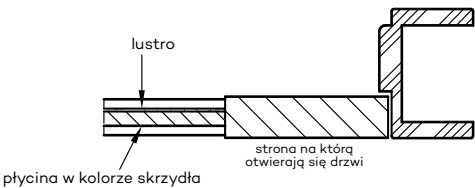
Drzwi ESTRA 10 bezprzylgowe lub przylgowe w wariantcie "Rewers"
