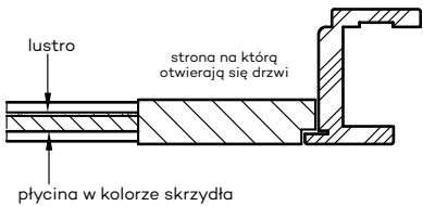
Drzwi ESTRA 10 z odwróconą przylgą w wariantcie "Rewers"
