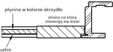
Drzwi ESTRA 10 z odwróconą przylgą w wariantcie "Rewers"
